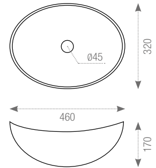
188277 Lavabo New Metal 46×32×17 cm./18.1"×12.6"×6.7" E250
