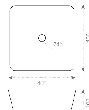
188753 Lavabo Legacy 40×40×10 cm./15.7"×15.7"×3.9" E450
